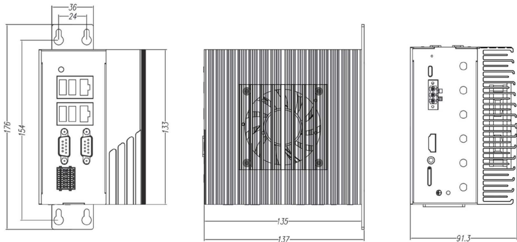
整机尺寸图
