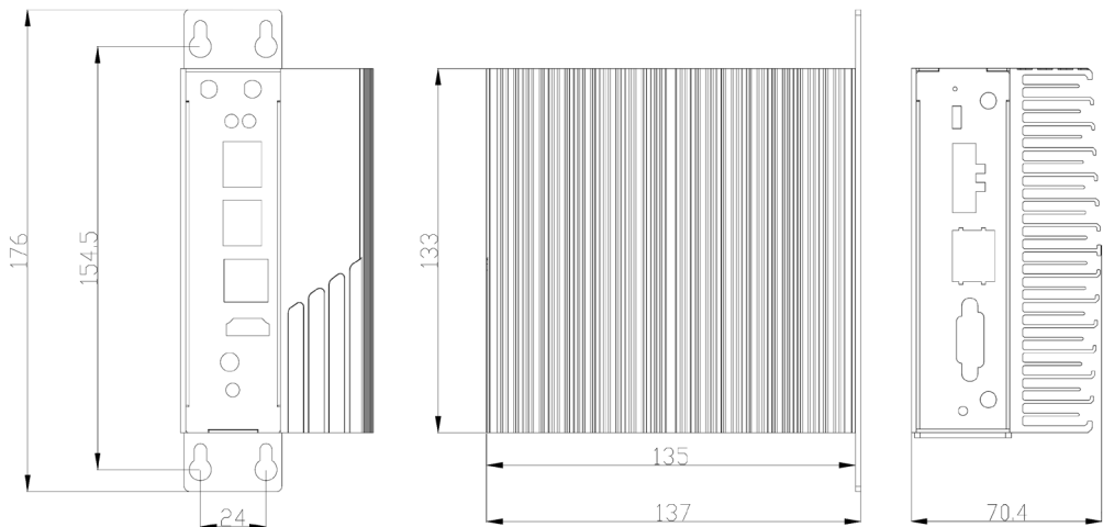
整机尺寸图
