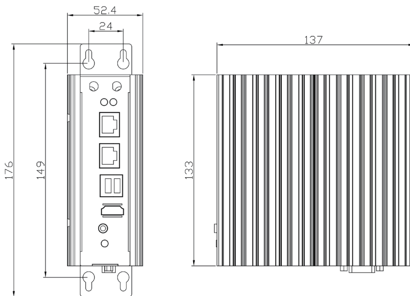
整机尺寸图
