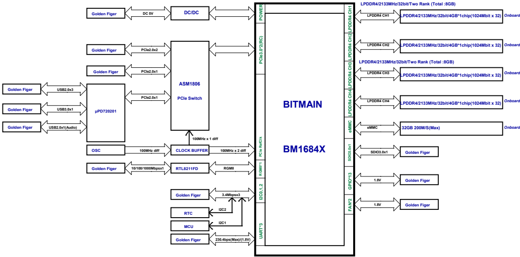
系统框图
